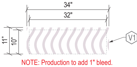
Window Vinyl 5 Layout QTY 4 Scale: 1/2" = 1'-0"
